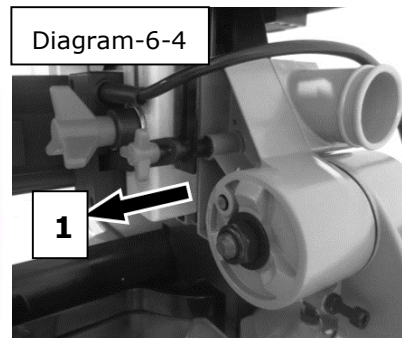
so lässt sich der Arretierbolzen (1) leicht aus der Bohrung ziehen und die Kappsäge schwenkt nach oben. (6-4)
